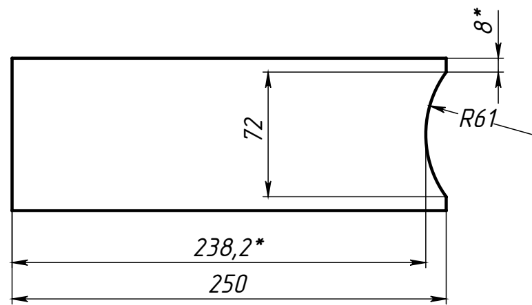
Поз.1 (Основание)
