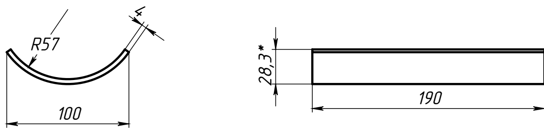
Поз.3 (Ложемент)
